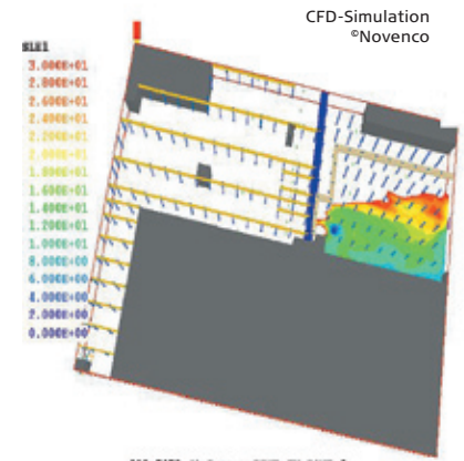
Rauchverhalten
